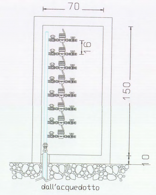
PARTICOLARE NICCHIA ALLOGGIAMENTO CONTATORI SCALA 1:25
