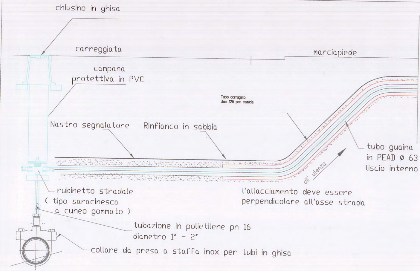
ALLACCIAMENTO TIPO: UTENZE ACQUEDOTTO SCALA 1:25
