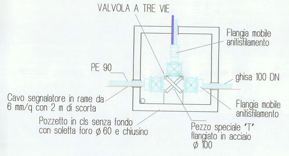
POZZETTO DI COLLEGAMENTO ACQUEDOTTO SCALA 1:50
