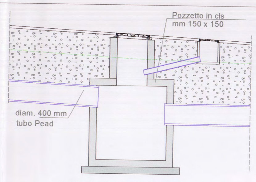
POZZETTO ALLACCIO ACQUE BIANCHE SCALA 1:50
